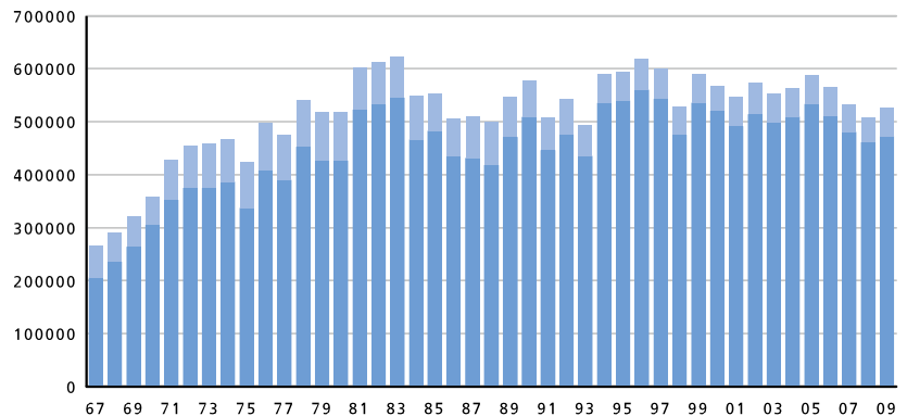
Eine halbe Million Wasservögel überwintern in der Schweiz. Dunkel: Wasservögel ohne Möwen; hell: Möwen.
