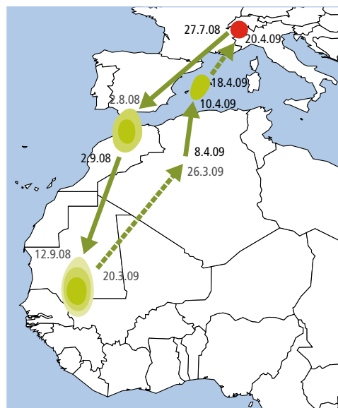
Unsere allerersten Ergebnisse von Geolocators zeigen den Vogelzug zweier Wiedehopfe aus dem Wallis nach Afrika und zurück (links Weibchen, rechts Männchen).
